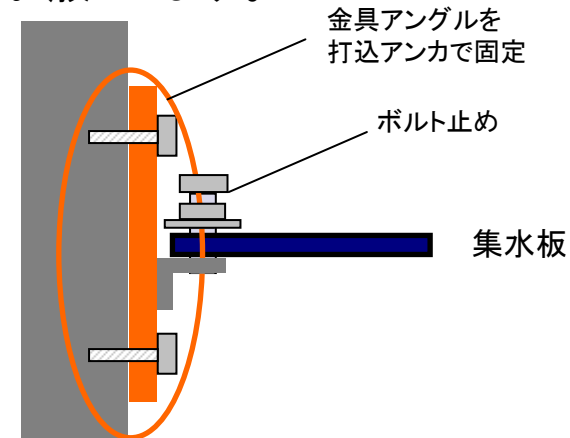
施工方法例
